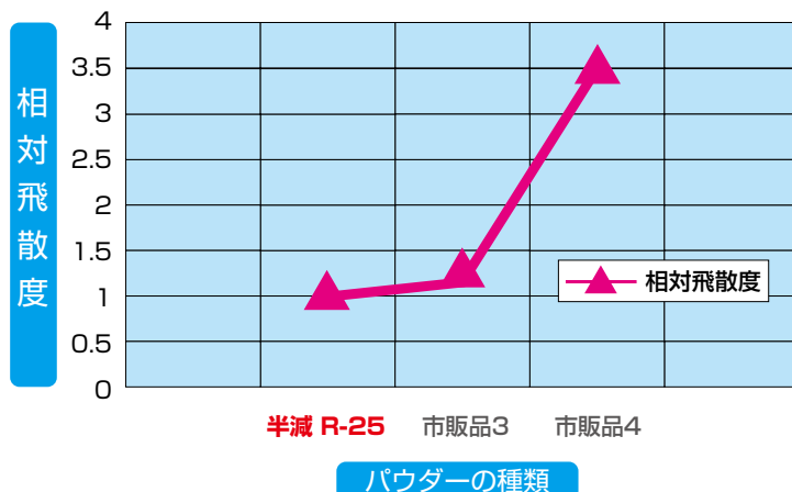
各社撥水性パウダーの相対飛散度／基準＝半減・R-25
